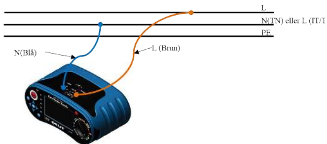
Figur 6.5.7 L-N Kortslutningsström och Z nät impedans – Koppling av testledningar PC-2 adaptorn för vägguttag kan också användas.
