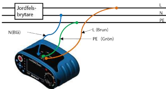
Figur 6.5.1 Inkoppling Z_{\text{LOOP}} med Jordfelsbrytare PC-2 Pluggadapter kan ocks användas
