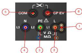
5.2 Ovansida (Ingångsterminal)
