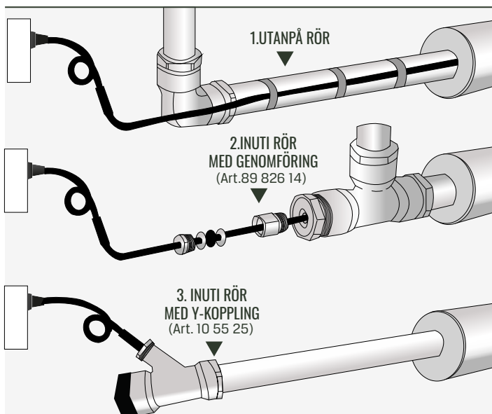
Art.89 826 14 Genomföring (bild 2) R 15/20 genomföring för invändig dragning av värmekabel i rör. Vattentät genomföring.
